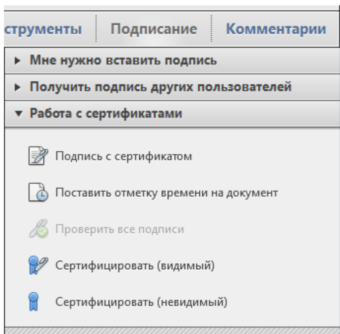
Рисунок 12. Добавление ЭП
