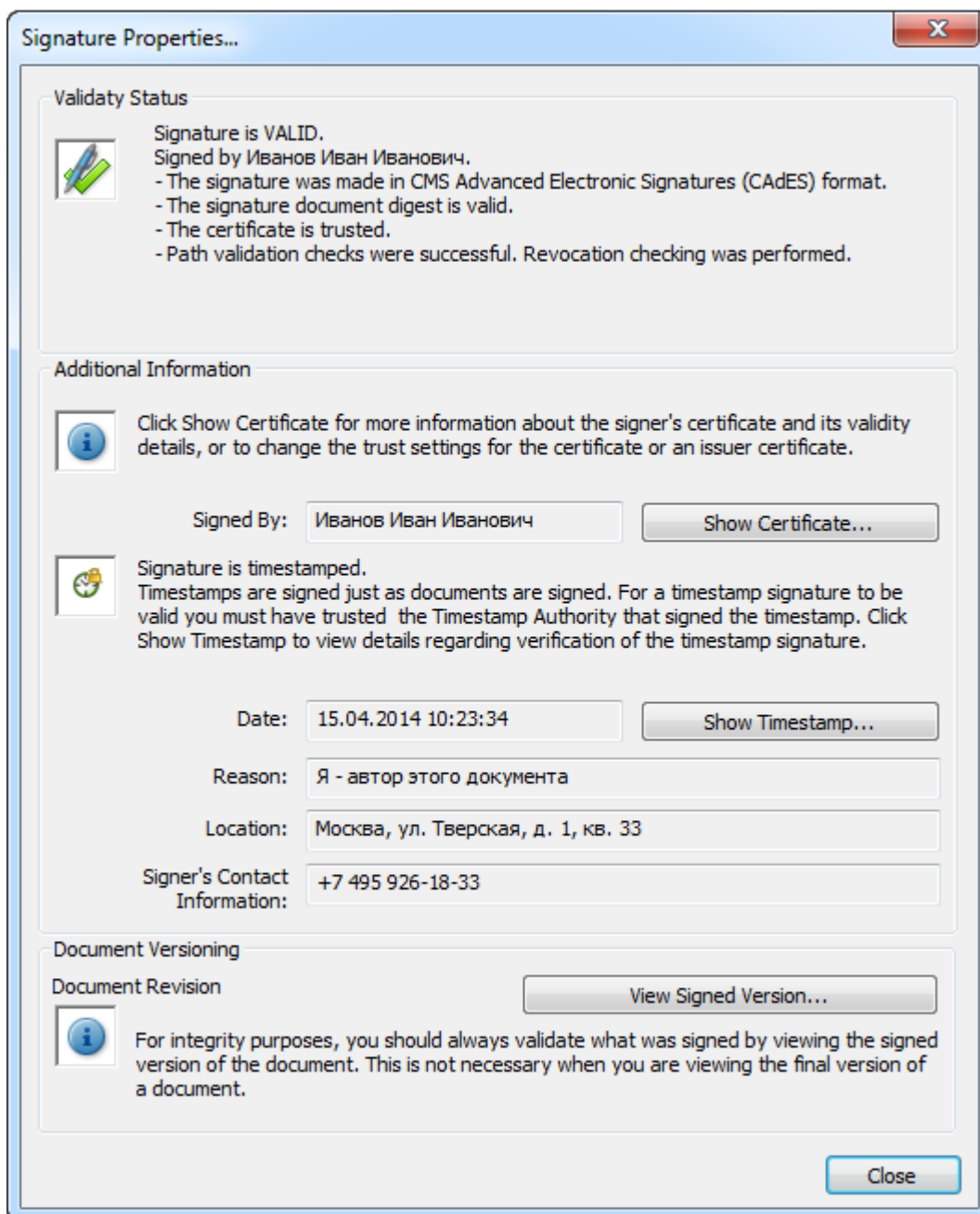
Рисунок 23. Параметры подписи
