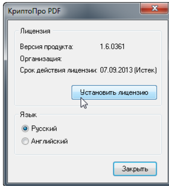
Рисунок 10. Панель настройки
